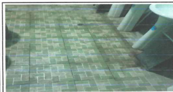
Foto 3: Sustrucción de piso de concreto con acabado liso por piso cerámico antideslizante, incluyendo preparación de superficie en baños de primer y segundo nivel.
